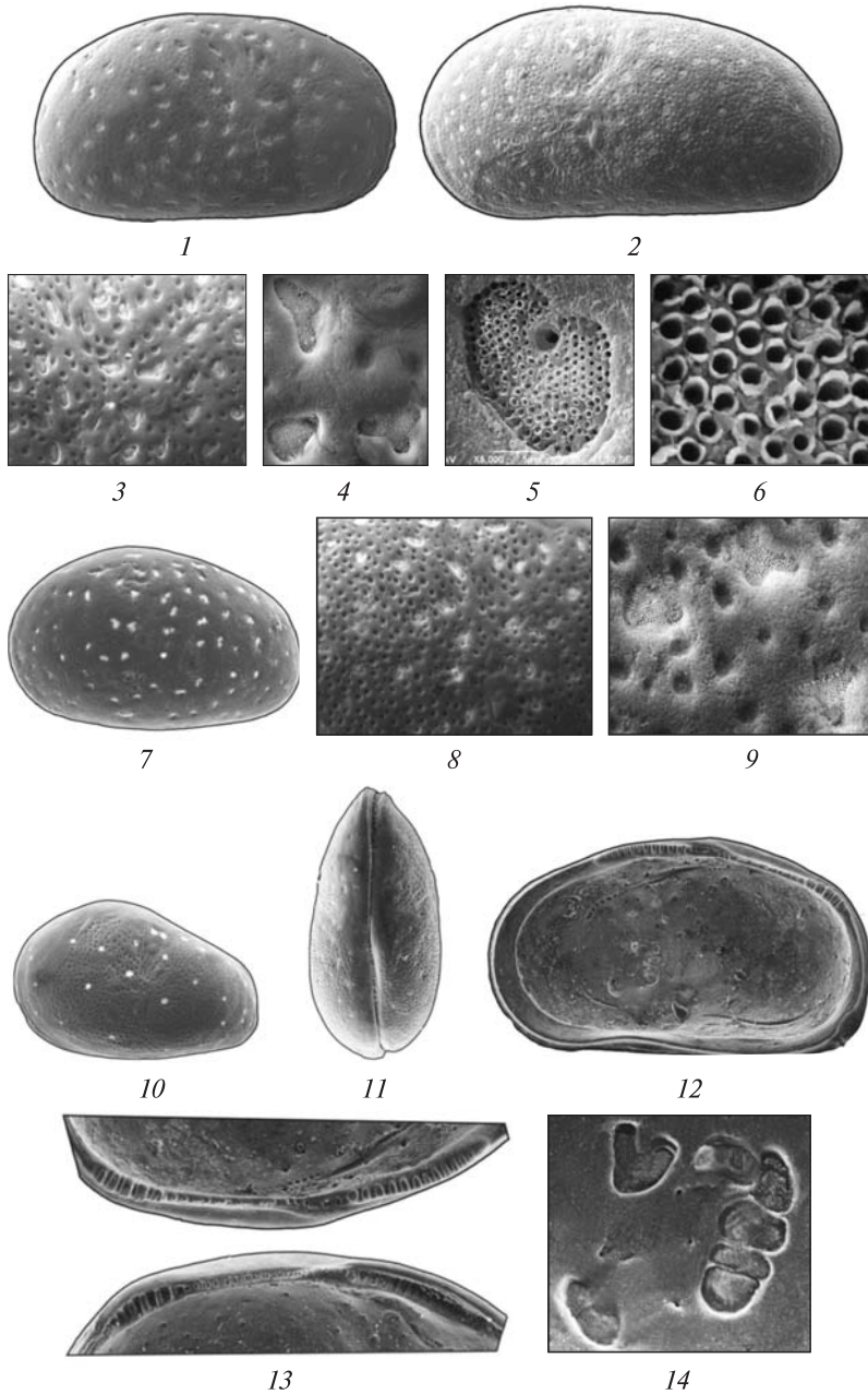
Рис. 3. Палеонтологическая таблица Cyprideis pontica Krstić, 1968: 1 — самка, ПС, взрослая особь с внешней стороны (×130), верхний сармат, северо-западный шельф Черного моря, скв. 67; 2 — самец, ЛС, взрослая особь с внешней стороны, (×95), нижний мэотис, северо-западный шельф Черного моря, скв. 55; 3 — фрагмент поверхности взрослой особи, самец (×250); 4 — поверхностные поры (×1000); 5 — ситовидная пластинка (×5000); 6 — внутренние поры (×13000); 7 — личинка средней стадии развития (×190), верхний мэотис, Таманский п-ов, разрез Попов Камень; 8 — фрагмент поверхности личинки (×250); 9 — поверхностные поры личинки (×1000); 10 — личинка ранней стадии развития (×230), нижний мэотис, Таманский п-ов, разрез Железный Рог; 11 — самка, вид сбоку (×140), нижний мэотис, северо-западный шельф Черного моря, скв. 55; 12 — самка, ПС, взрослая особь с внутренней стороны (×120), неоплейстоцен, посткарангат, северо-западный шельф Черного моря, скв. 350; 13 — замок (×180); 14 — мускульные отпечатки (×600)
