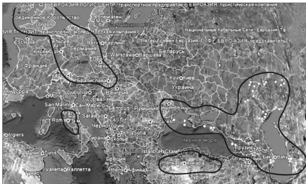
Рис. 5. Карта ареалов Cyprideis pontica Krstić и Cyprideis torosa (Jones) в Паратетисе и Средиземноморском бассейне (средний миоцен-плиоцен)
