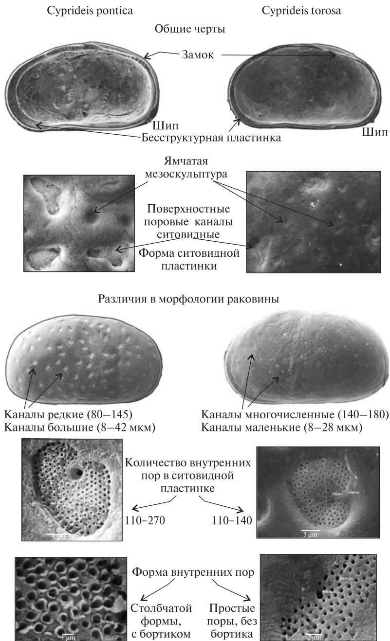
Рис. 4. Сравнение морфологии раковины Cyprideis pontica Krstić и материнского вида Cyprideis torosa (Jones)
