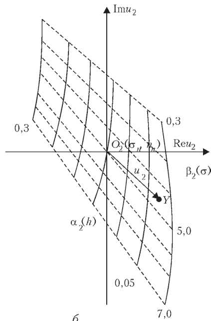
Годографы информационных сигналов системы ВТП–МОС при изменении параметров ОК на частоте \omega_1 ( a ) и \omega_2 ( б )
