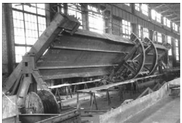
Рис. 4. Длинная балка в кантователе
