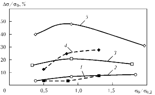
Рис. 3. Влияние величины относительной нагрузки \sigma_0/\sigma_{0,2} для образцов из стали Ст3 (1, 4) и сплава АМгб (2, 3, 5) на эффективность ЭДО при различной запасенной энергии заряда: 1 — E = 300 Дж; 2 — 130; 3 — 300; 4 — 800; 5 — 800
