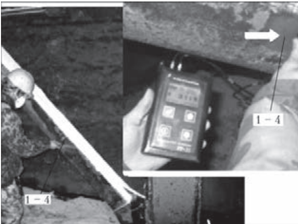
Рис. 5. Местные утонения металла стенок вертикальных связей из замкнутого коробчатого профиля вследствие внутренней коррозии (1-4) (потеря сечения от проектного значения 22 %)
