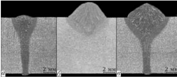
Рис. 2. Макрошлифы проплавлений, выполненных лазерной сваркой (а), сваркой МАГ (б) и гибридной лазерной сваркой + сваркой МАГ (в) [21]
