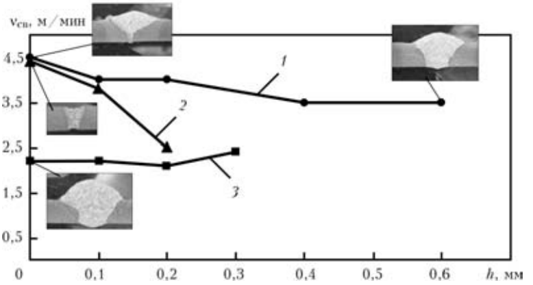
Рис. 4. Влияние ширины h зазора на максимальную скорость v_{св} гибридной сварки (1) (мощность CO_2 -лазера 2250 Вт), лазерной сваркой (2) и сваркой МИГ (3) (мощность 9 кВт) (сплав СМп250 толщиной 2,13 мм) [25]
