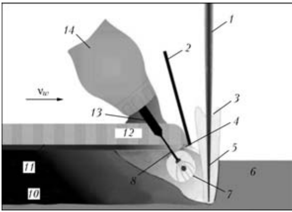
Рис. 12. Схема гибридной лазерно-дуговой сварки под флюсом [28]: 1 — лазерный пучок; 2 — разделительная пластина; 3 — плазмоиспарение металла; 4 — жидкий шлак; 5 — парогазовый канал; 6 — основной металл; 7 — раковина в дуговом шве; 8 — электродная проволока для дуговой сварки под флюсом; 9 — расплавленная ванна; 10 — металл шва; 11 — твердый шлак; 12 — флюс; 13 — мундштук; 14 — бункер для флюса
