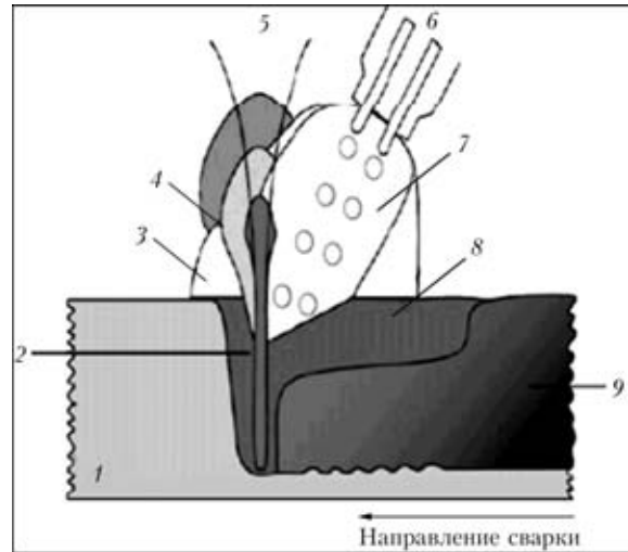
Рис. 11. Схема лазерной тандем-сварки [9]: 1 — обрабатываемое изделие; 2 — парогазовый канал; 3 — облако защитного газа; 4 — индуцированная лазером плазма; 5 — лазерный пучок; 6 — электрод; 7 — дуга; 8 — наплавленный валик; 9 — сварочная ванна
