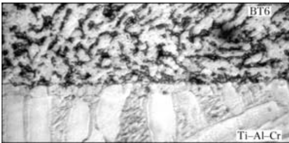
Рис. 6. Микроструктура ( \times 1250 ) зоны контакта сварного соединения алюминид титана+VT6
