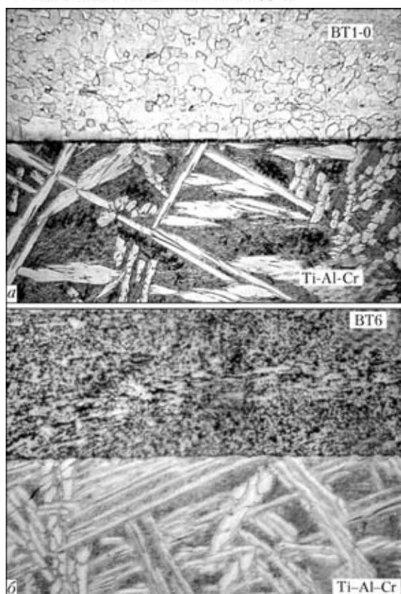
Рис. 1. Микроструктура зон контакта сварного соединения алюминид титана с техническим титаном BT1-0 (а, \times 100 ) и сплавом VT6 (б, \times 200 )
