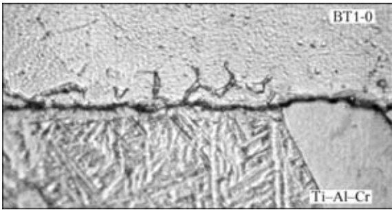
Рис. 4. Микроструктура ( \times 1250 ) диффузионной зоны с зернограничной диффузией алюминия в титан
