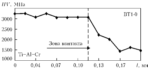
Рис. 5. Распределение микротвердости в зоне контакта сварного соединения алюминид титана+VT1-0 ( l — расстояние между уколами индентора)
