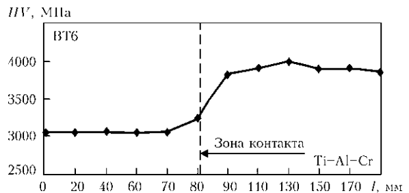
Рис. 8. Распределение микротвердости в зоне контакта сварного соединения алюминид титана+VT6
