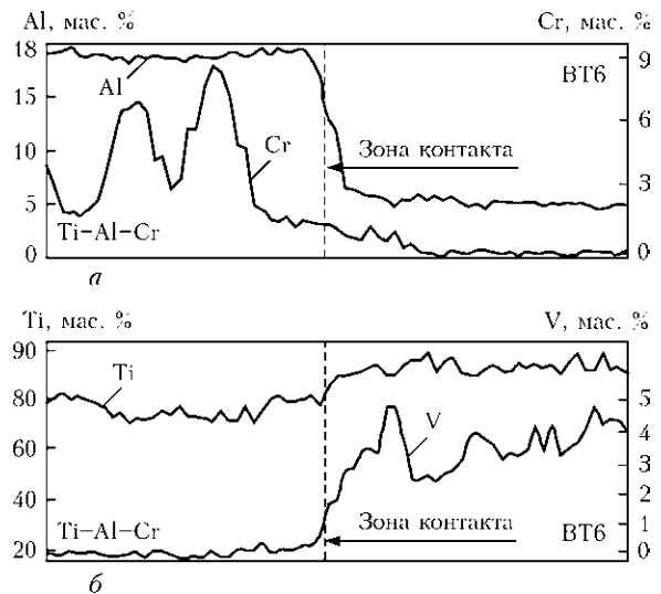
Рис. 7. Распределение алюминия, хрома (а) и титана, ванадия (б) в зоне контакта сварного соединения алюминид титана+VT6
