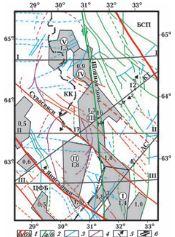
Рис. 21. Трехмерная магнитная модель средней и нижней коры центральной части Карельского кратона: 1 — система разломов северо-западного простирания (а — I, б — II, в — III рангов); 2 — система разломов меридионального шва (а — II, б — III рангов); 3 — разломы других направлений; 4 — дугообразные разломы; 5 — направления падения разломов; 6 — направления горизонтальных перемещений. БСП — Беломорский складчатый пояс. Разрывные нарушения (сплошные линии — разломы, выделенные по геологическим данным, пунктирные — по магнитному и гравитационному полям). Другие условные обозначения см. на рис. 2, 3.
