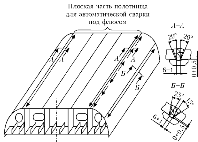
Рис. 3. Схема сварки внешней обшивки днищевых секций судна: длинная стрелка — направление сварки пазов; короткая — корневых проходов швов на ФКП
