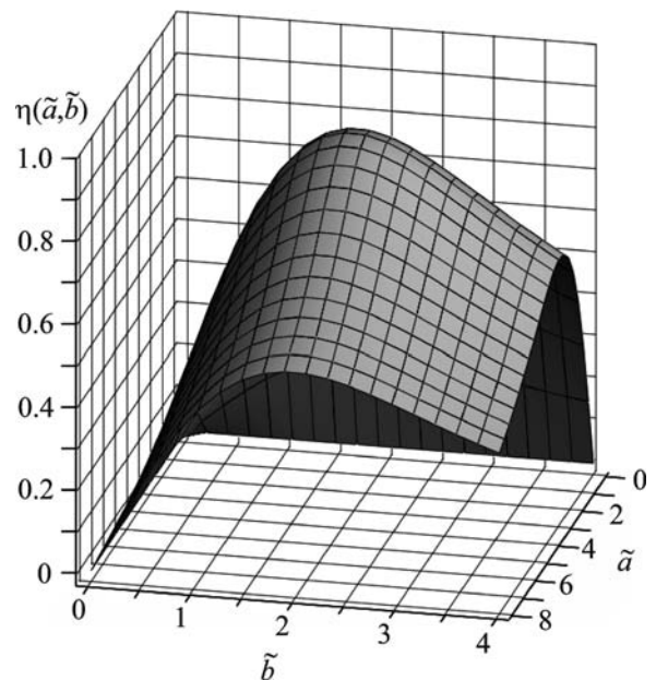
Рис. 2. Эффективность возбуждения волны TE_{10} в прямоугольном волноводе при изменении его поперечных размеров
