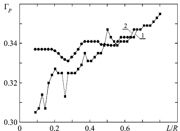
Рис. 5. Зависимости коэффициента отражения \Gamma_p от расстояния между зеркалами L/R для основного колебания в полусферическом ОР (кривая 1) и резонаторе с отрезком сверхразмерного волновода при наличии дифракционной решетки (кривая 2)
