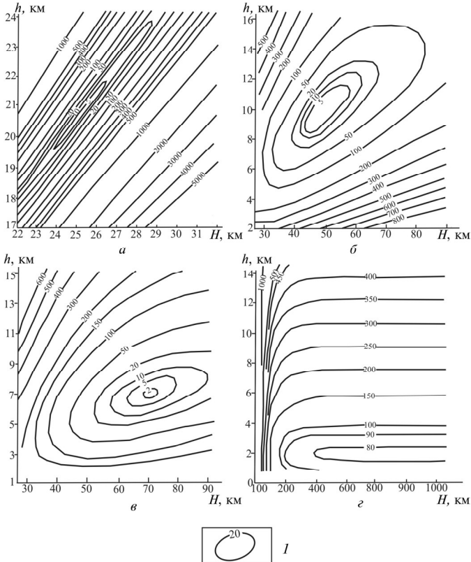
Рис. 1. Модель МП-1. Рельеф структуры целевого функционала в различных плоскостях I_z = \text{const} сечений пространства параметров h-H-I_z : а - I_z = 1200 \cdot 10^{-2} А/м; б - I_z = 160 \cdot 10^{-2} А/м; в - I_z = 120 \cdot 10^{-2} А/м; г - I_z = 70 \cdot 10^{-2} А/м; 1 - линии рельефа целевого функционала
